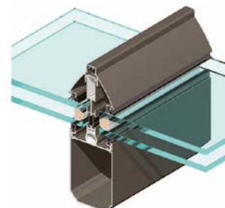
Chevron TOURMALINE, avec capot intérieur rapporté en option.
